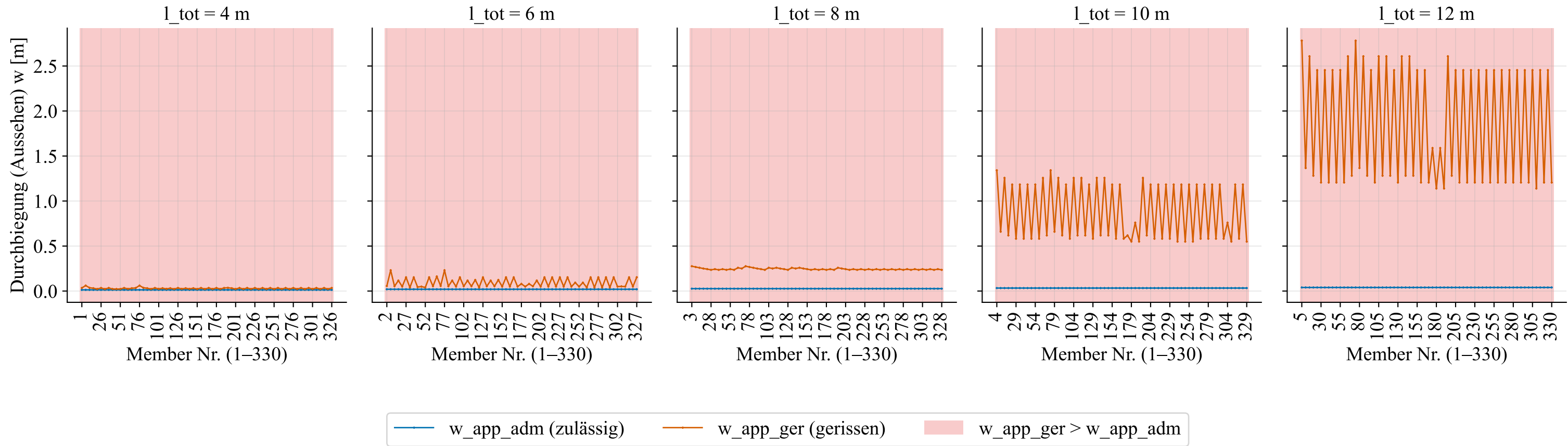
Durchbiegung w_app_adm (zulässig) vs. w_app_ger (gerissen) je Member, kategorisiert nach Spannweite (Members_rc_rib_simple_)
